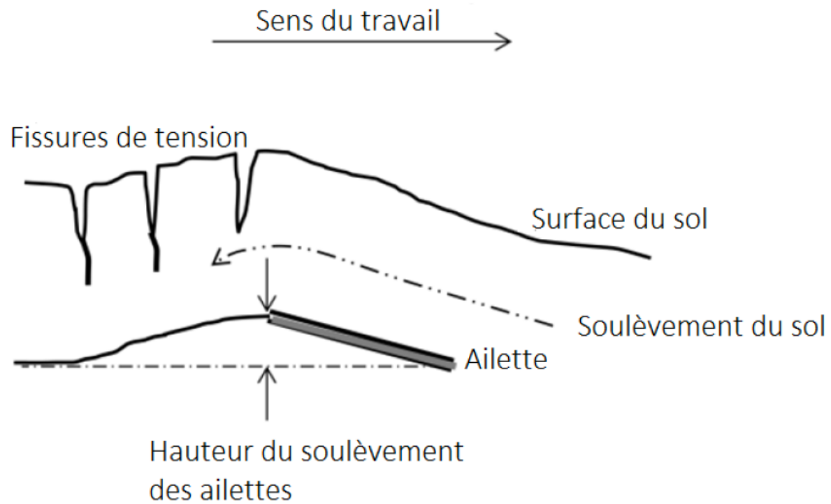
Soulèvement du sol occasionnant des fissures par tension
