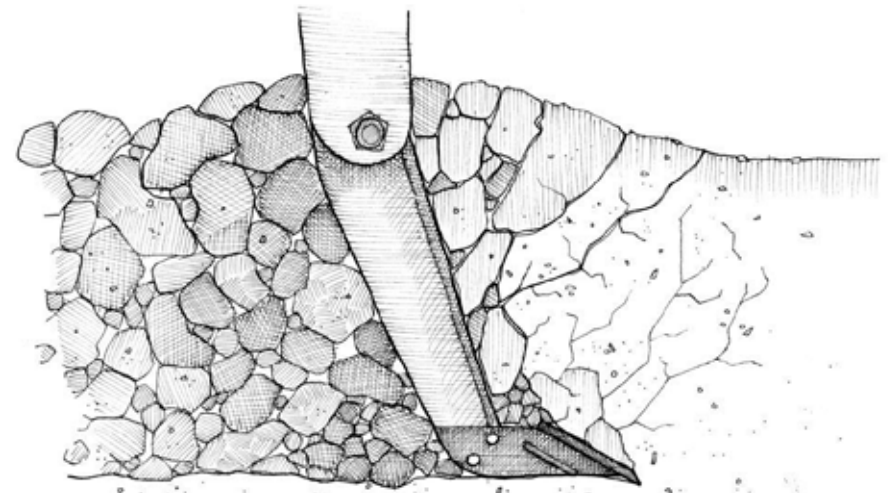
Fissuration par compression du sol exercée principalement par le socle - Cas de la sous-soleuse de Phacelia
