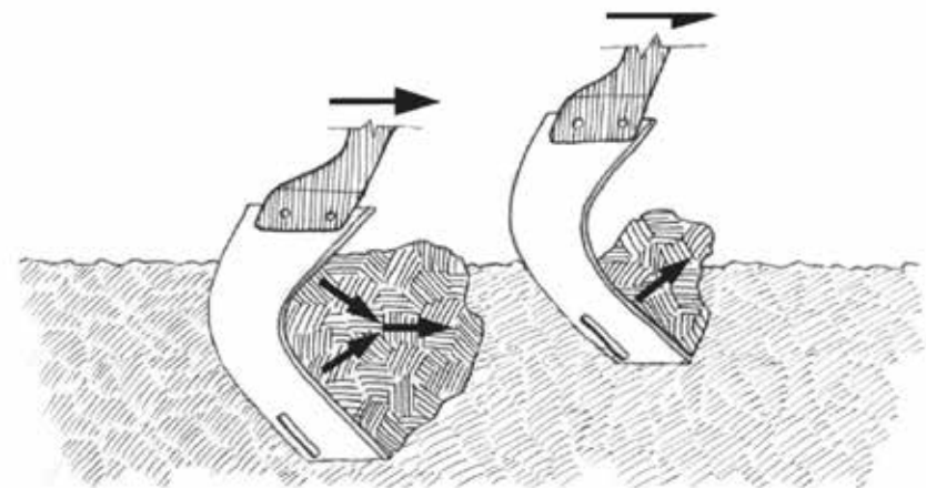
Profondeur trop importante qui augmente la compaction et la puissance
